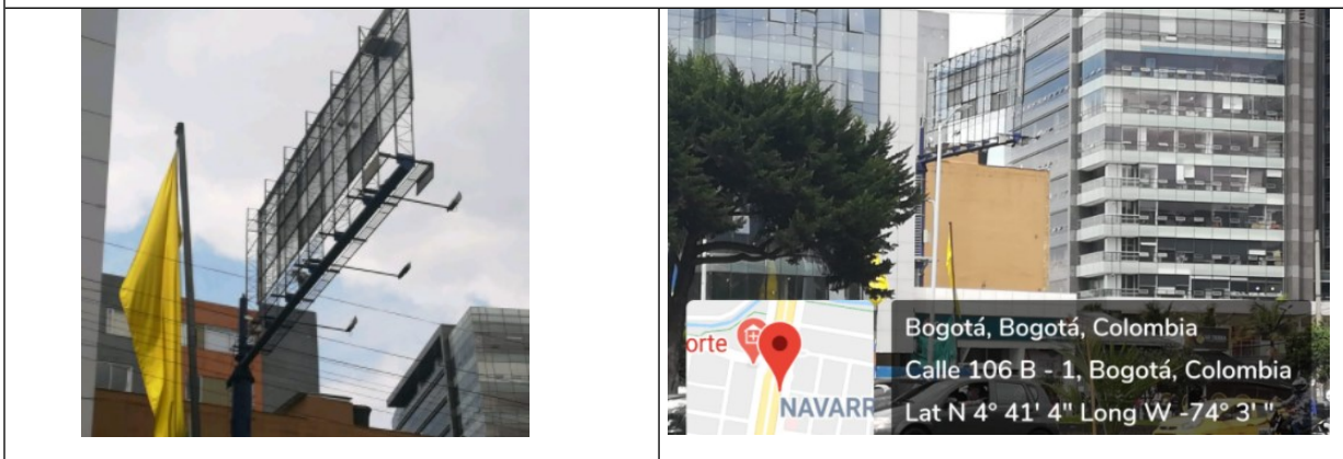
Foto 2. Detalle del tablero desmontado de la estructura de la valla ubicada en la Calle 108 N° 45 - 27 orientación Sur - Norte
